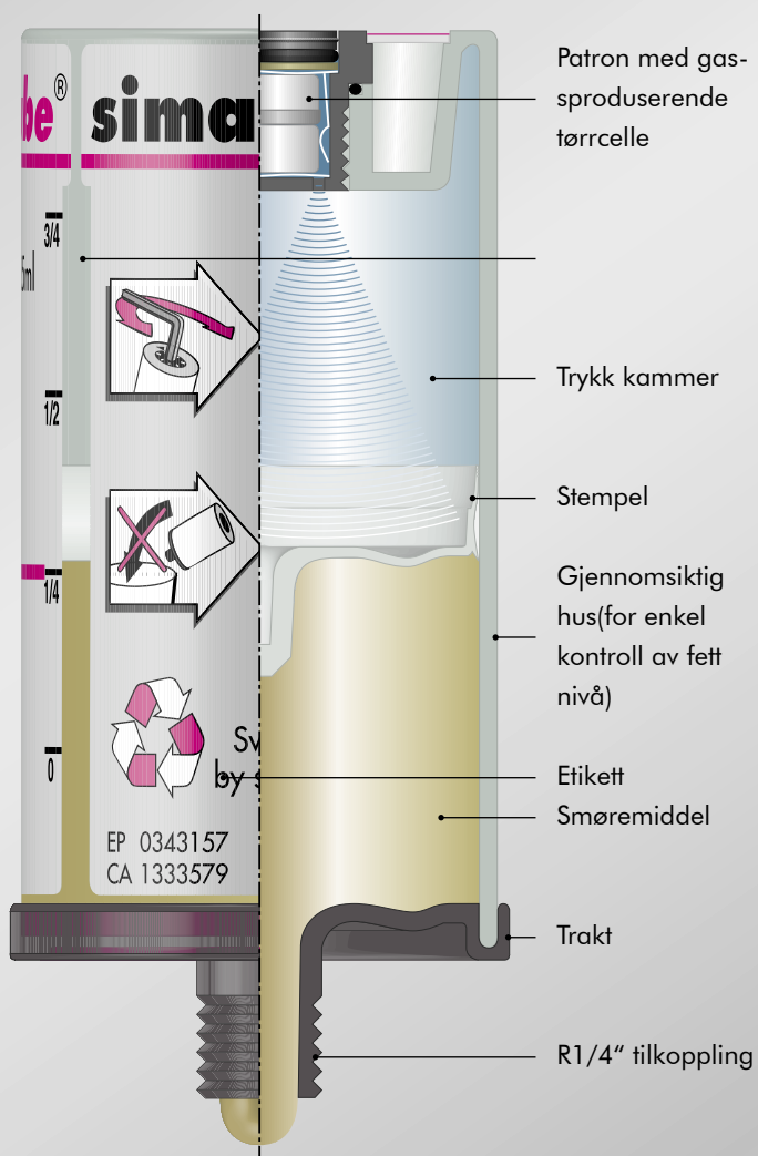
Patron med gassproduserende tørrcelle
